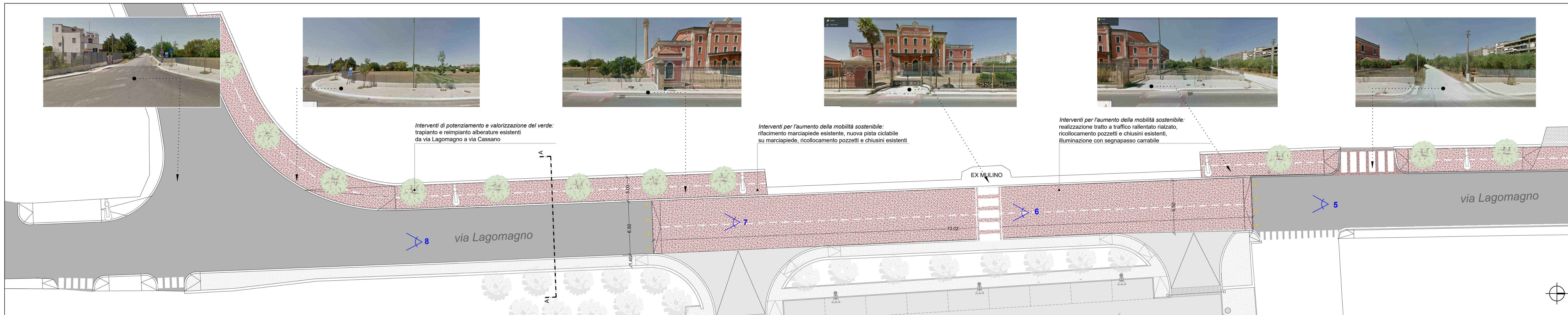
TRATTO B - scala 1:200
