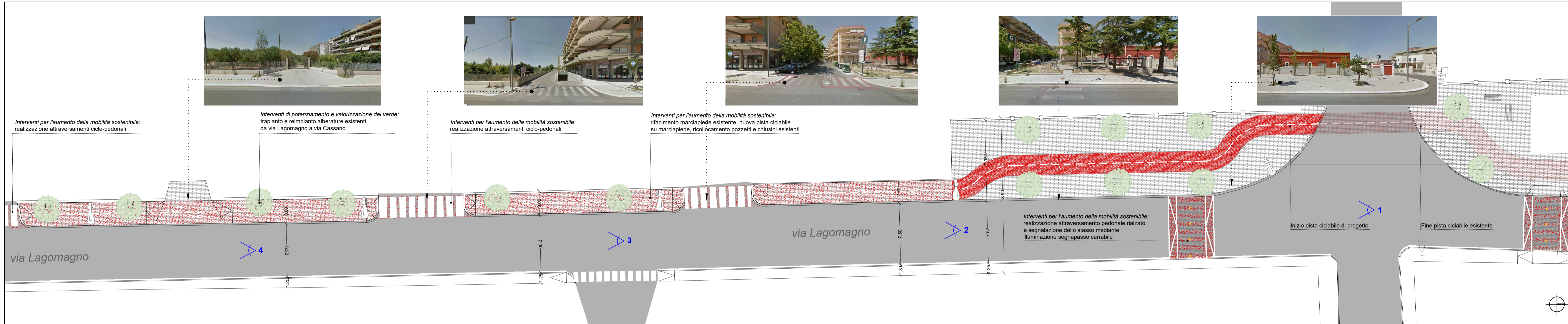
TRATTO A - scala 1:200
