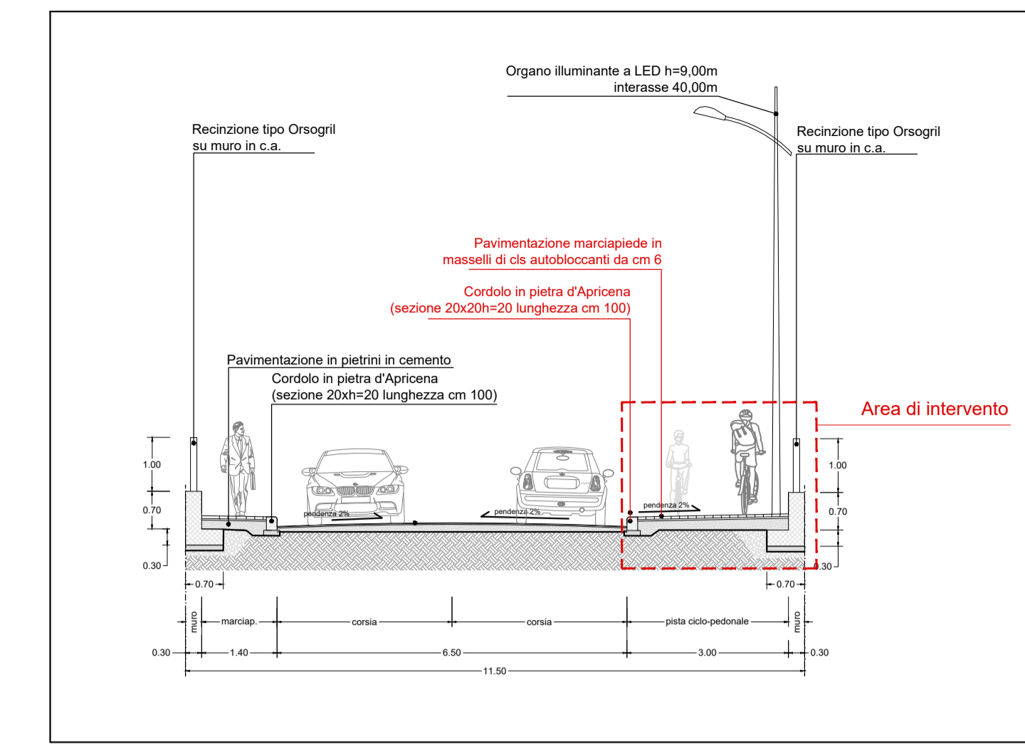
SEZIONE AA' - scala 1:200
